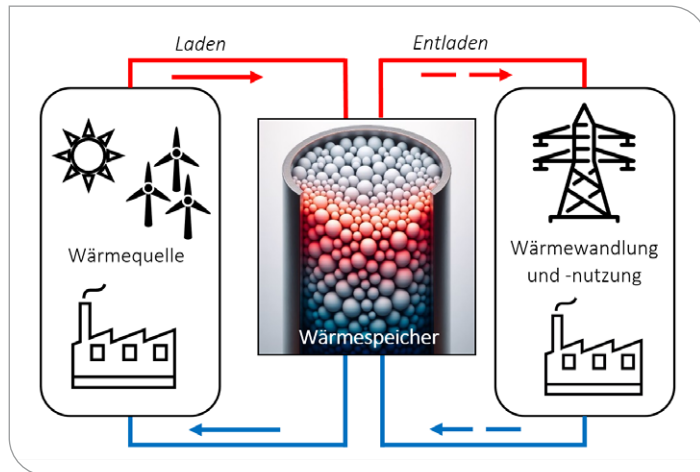
Nutzung eines Hochtemperatur-Wärmespeichers zur Bereitstellung von Prozesswärme oder Strom. (Grafik: KIT/KALLA)
