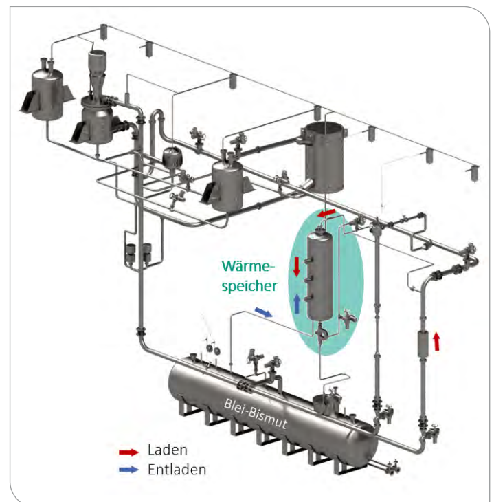
Test eines Pilotspeichers im Blei-Bismut-Kreislauf am KALLA. (Grafik: KIT/Daubner)
